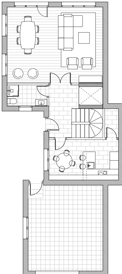
PLANTA BAJA
